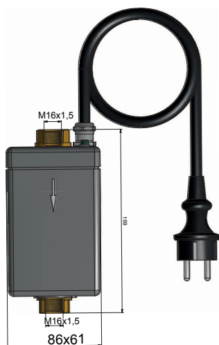
GGP250 B M16X1,5F M16X1,5F TYPE C
